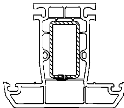
Импост 82 мм Арт. 39211.00
