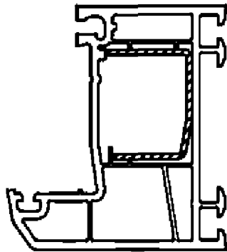
Рама 63 мм Арт. 39071.00
